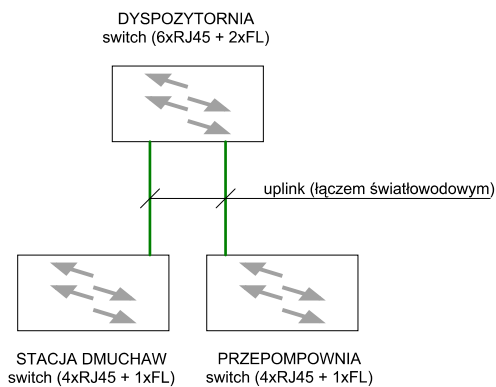
struktura połączeń urządzeń aktywnych w sieci ethernet
